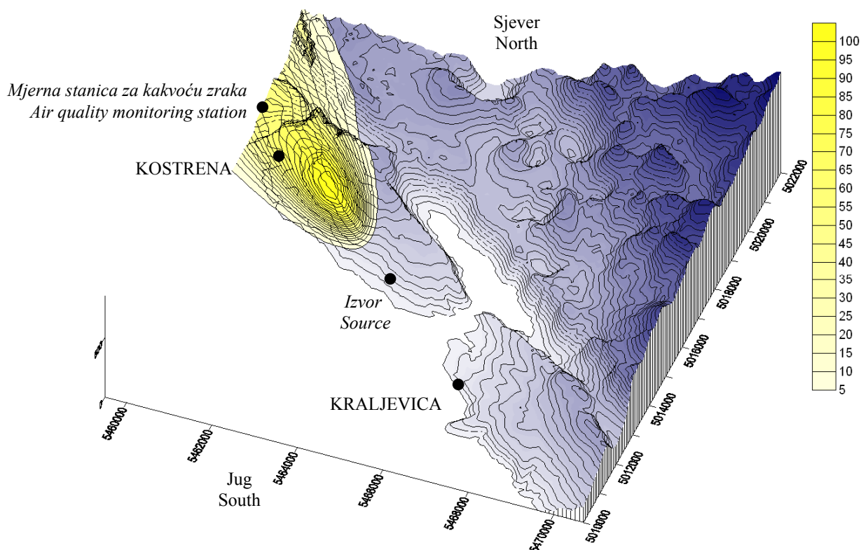
Slika 4. Konturni prikaz površinske koncentracije SO_2 ( \mu g/m^3 ) za odabranu domenu i vrijeme (9.7.2006. 19:00) Figure 4. 3D contour plot of SO_2 ground concentrations ( \mu g/m^3 ) on the 9 th June 2006. at 19h
